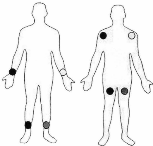
Derivaciones de Bipolares y Unipolares
